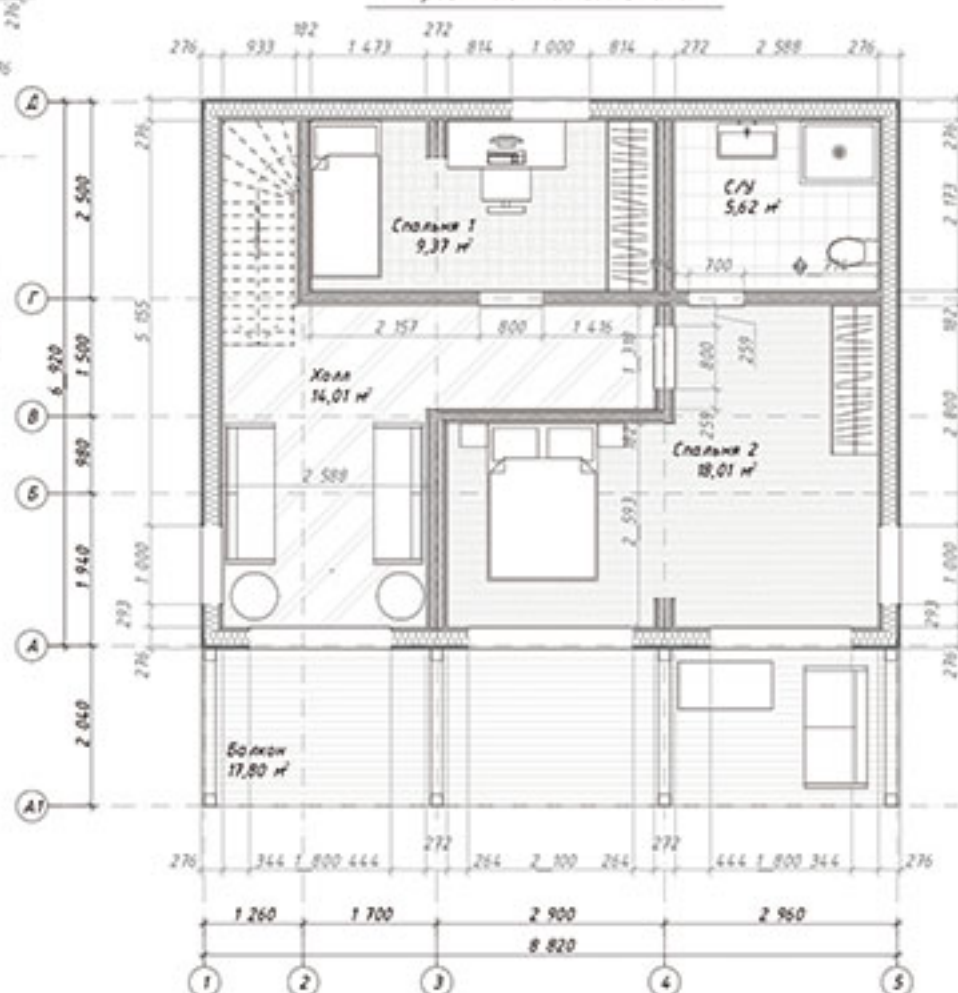
Проектный план 2го этажа
