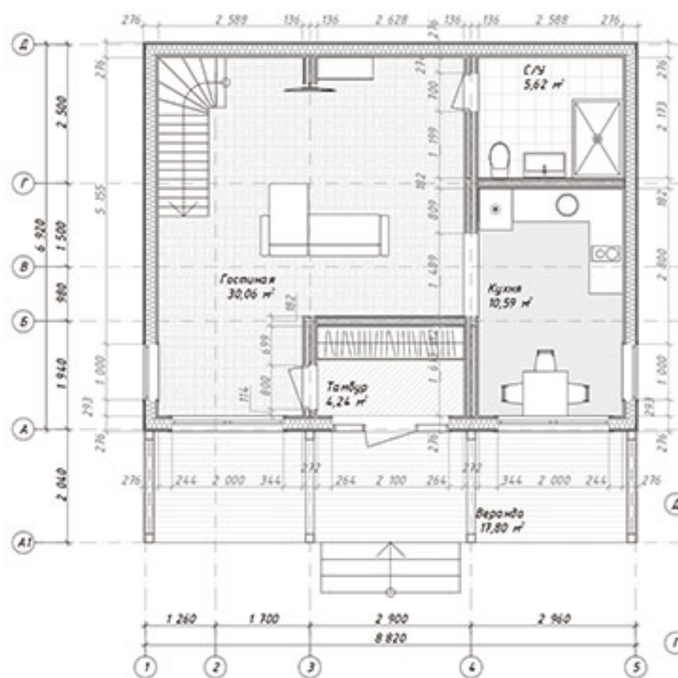
Проектный план 1го этажа
