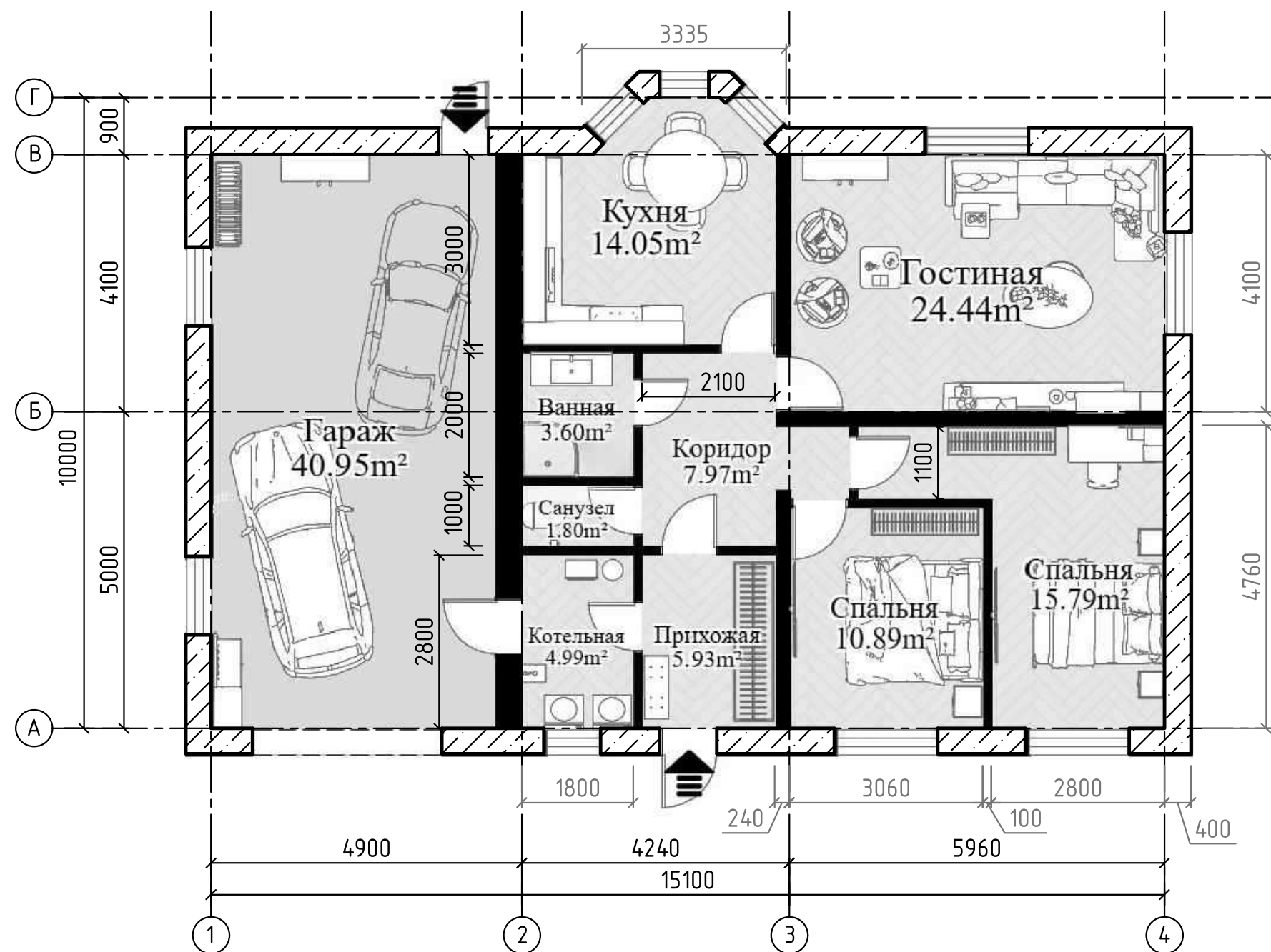
Экспликация помещений
